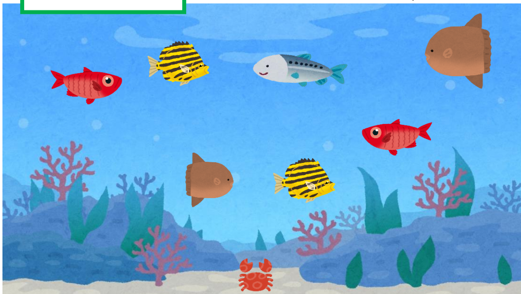
イメージ図
